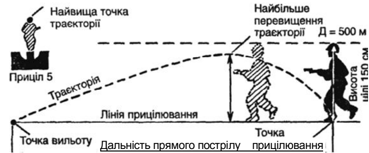
Мал. 48. Прямий постріл
