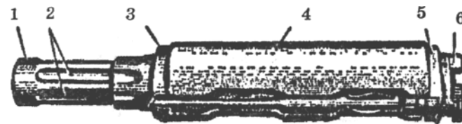
Мал. 24. Газова трубка із ствольною накладкою: 1 - газова трубка; 2 - напрямні ребра для газового поршня; 3 - передня з'єднувальна муфта; 4 - ствольна накладдка; 5 - задня з'єднувальна муфта; 6 - виступ
