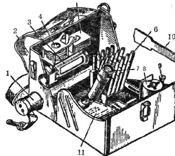
Мал. 156. Військовий прилад хімічної розвідки (ВПХР):
